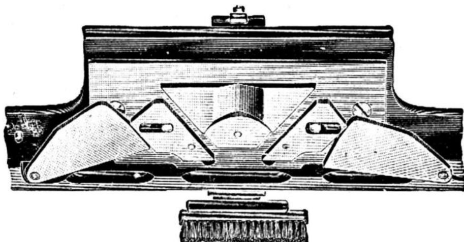
Randschloss bei Exzeterschloss (auch Rechts und Rechts-Apparat genannt.)
