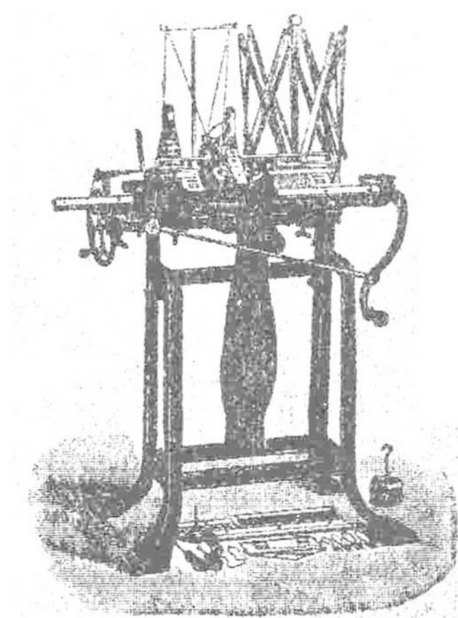
Strickmaschine mit kurzem Schlitten u. Schlauchschloß
