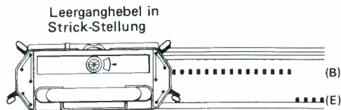
Fig.61 Nadelrückholer in Position "2" schieben
